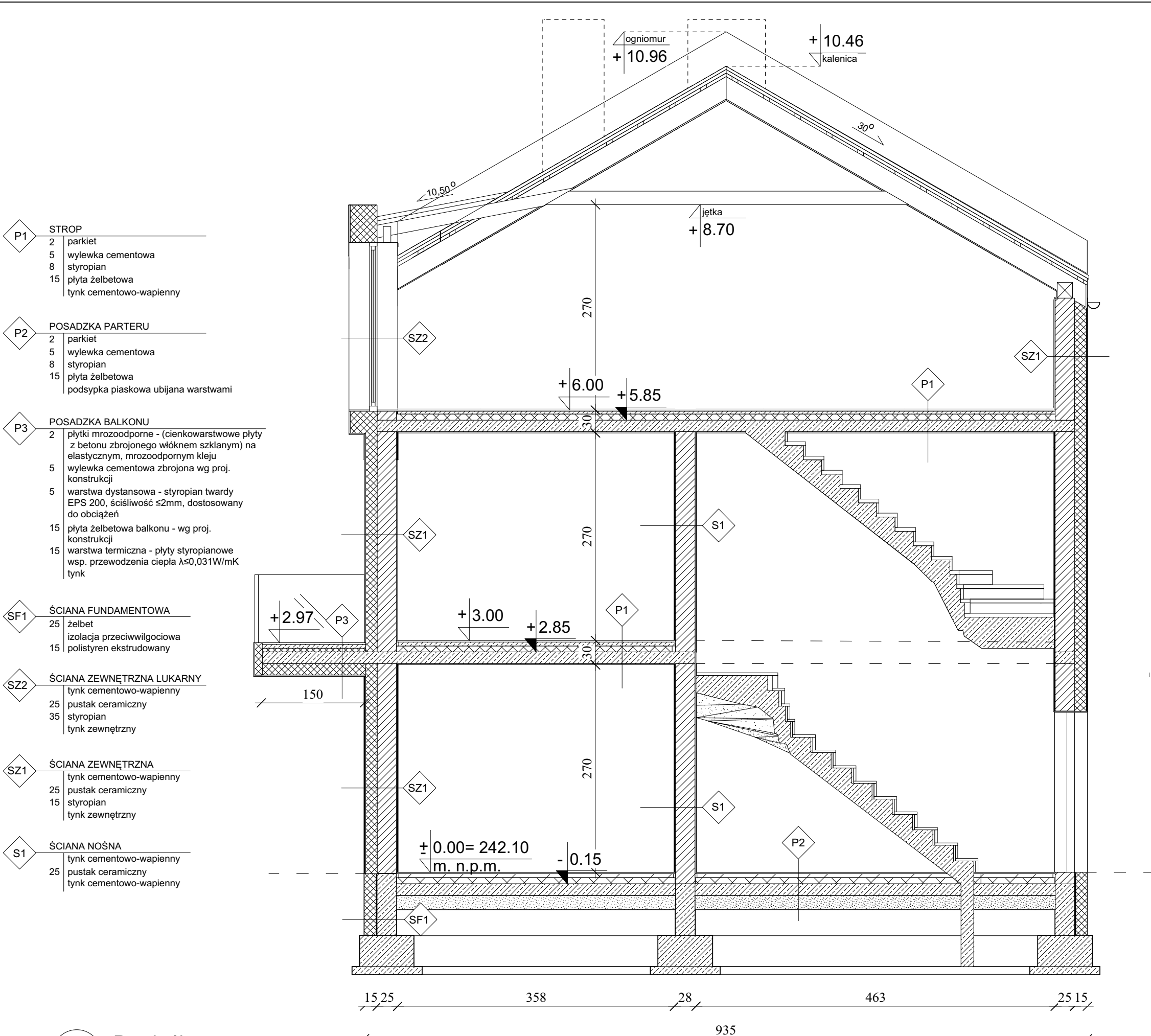
A-105 Przekrój Skala 1:50
